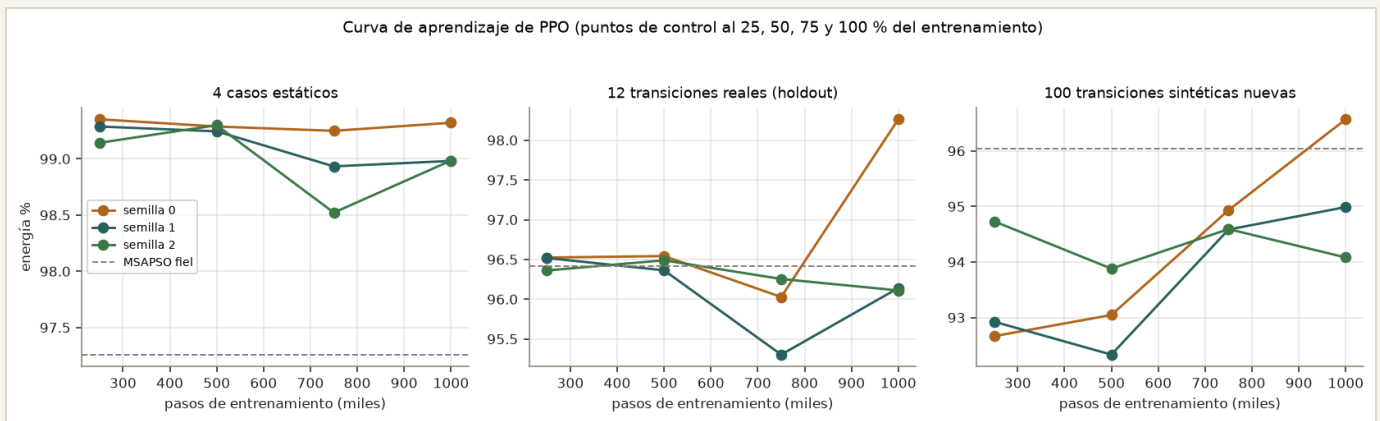
Figura G. Curva de aprendizaje de PPO por semilla (energía % en los tres conjuntos de prueba vs pasos de entrenamiento) y referencia del MSAPSO fiel.
