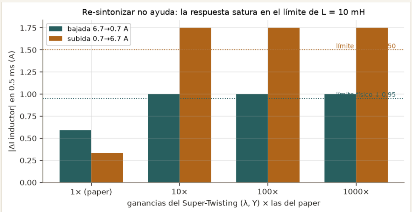
Figura D. Re-sintonizar el Super-Twisting: con ganancias \times 10 el convertidor ya satura en su límite físico; \times 100 y \times 1000 no mejoran (Caso 1, escalón 6.7 \leftrightarrow 0.7 A).
