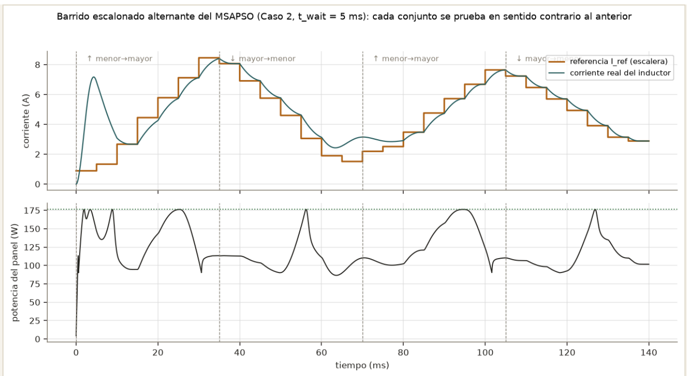
Figura B. Barrido escalonado alternante (Caso 2, t_{\text{wait}} = 5 \text{ ms} ): un conjunto se prueba de menor a mayor corriente, el siguiente de mayor a menor. Se muestra la referencia I_{\text{ref}} (escalera), la corriente real del inductor que entrega el Super-Twisting simulado y la potencia del panel.
