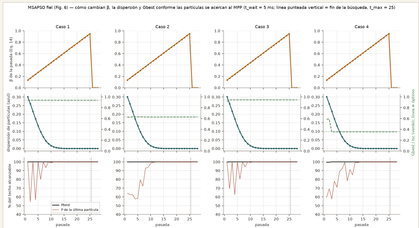
Figura A. MSAPSO fiel: \beta (Eq. 14), dispersión de las partículas, Gbest y potencia por pasada, en los 4 casos reales ( t_{wait} = 5 ms). Responde a la petición de graficar \beta conforme las partículas se acercan al MPP: Gbest se fija en las 1–3 primeras pasadas y la dispersión llega a \sim 0 hacia la pasada 12; de la 13 a la 25 el enjambre está colapsado.
