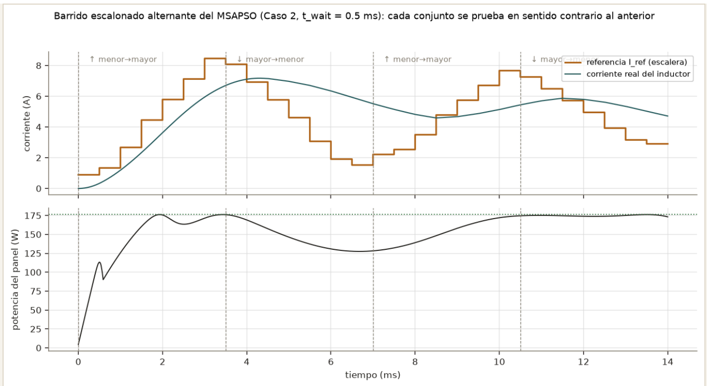
Figura C. Mismo barrido con t_{\text{wait}} = 0.5 ms: la corriente del inductor no alcanza a seguir los escalones (el convertidor está limitado por la pendiente de corriente con L = 10 mH).
