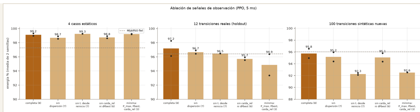
Figura J. Ablación de señales de observación (PPO, 5 ms; media de 2 semillas; puntos = semillas).
