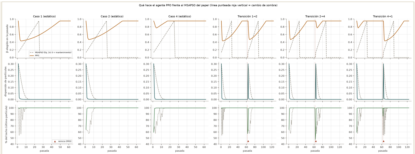
Figura F. Qué hace el agente PPO (semilla 0) frente al MSAPSO del paper: \beta elegido por pasada, dispersión de partículas, reinicios y potencia, en tres casos estáticos y tres transiciones.
