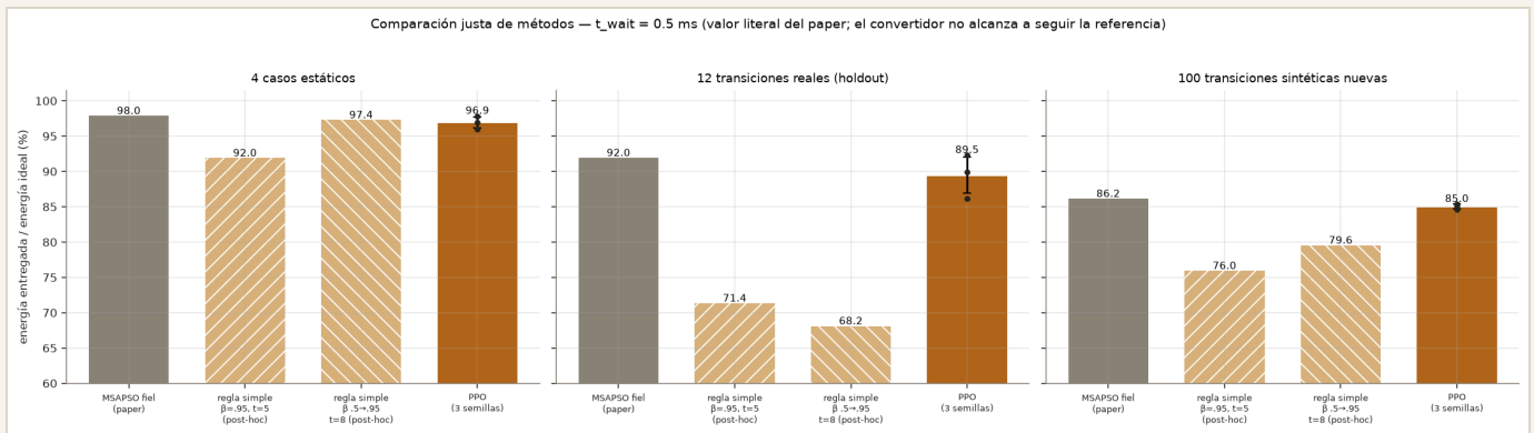
Figura I. Comparación en el régimen literal del paper ( t_{\text{wait}} = 0.5 ms).
