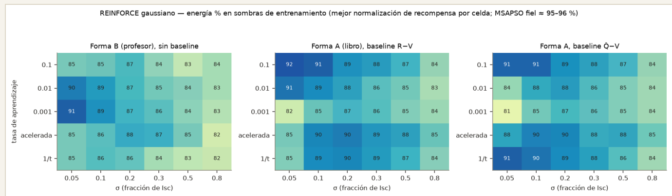
Figura E. REINFORCE gaussiano: energía % en sombras de entrenamiento según tasa de aprendizaje y \sigma (mejor normalización de recompensa por celda). La región buena es \sigma pequeña con paso efectivo c = lr/\sigma^2 moderado (0.3–1).
